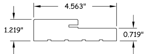
SIDE JAMB
