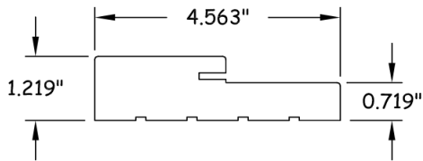
HEAD JAMB
